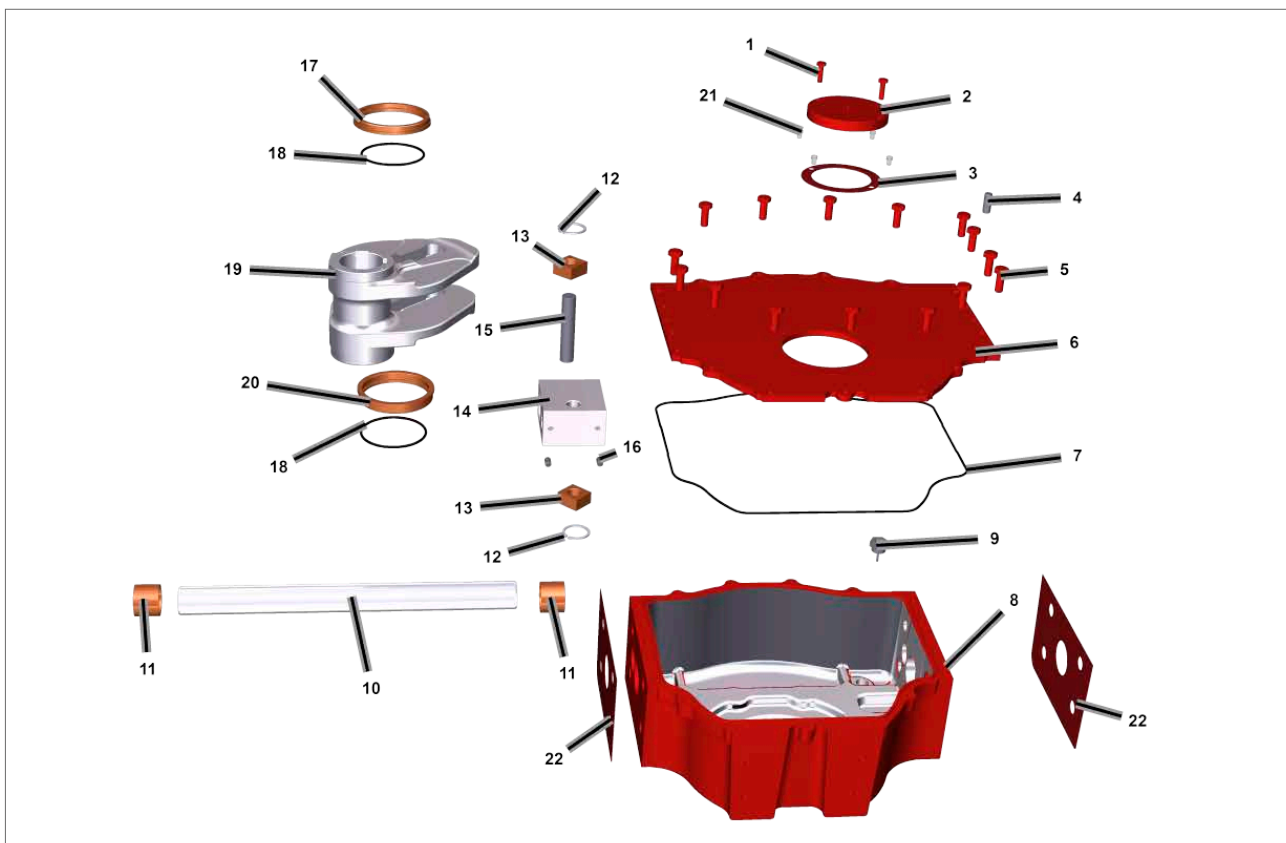
Fig 17.2 Midterkrop (støbejern) (Aktuator størrelse 130)
