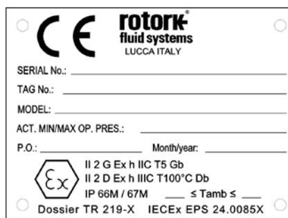
Fig 3.1 Aktuator IECEx navneskilt
