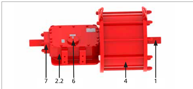
Fig 12.4 GPID (svejset krop) hovedkomponenter
