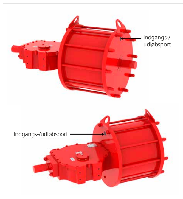
Fig 12.16 Udløbsport til dobbeltvirkende aktuator
