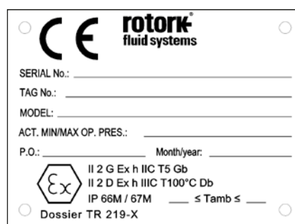
Fig 5.1 Aktuator ATEX navneskilt
