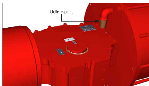
Fig 12.15 Udløbsport til enkeltvirkende aktuator
